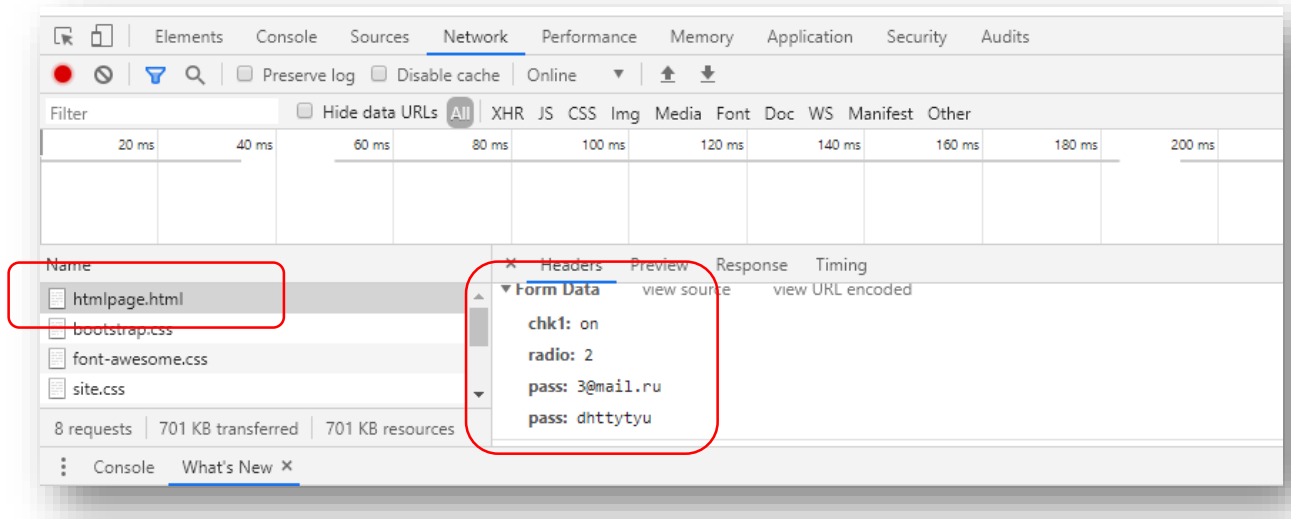
Рисунок 11 Режим разработчика
